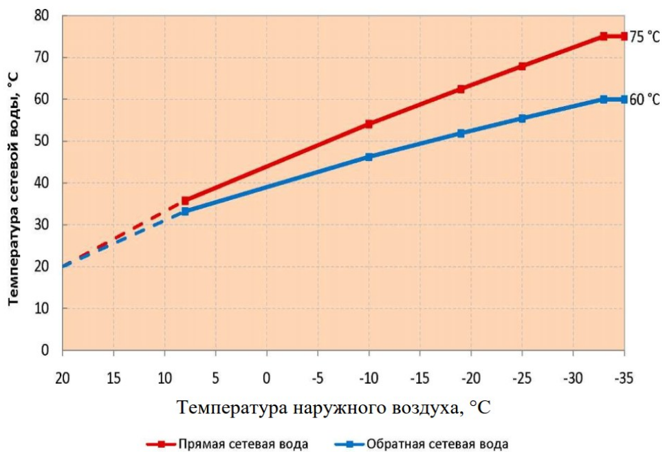
Рисунок 9 – Температурный график Котельной д. Даниловка, Котельной СДК (с. Паломохино, ул. Кирова, 28), Котельной (ж/д ст. Староверчская)
